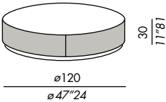
tavolo basso / low table TB-120R
