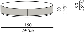
tavolo basso / low table TB-150900V
